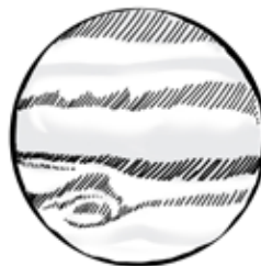
Jupiter
