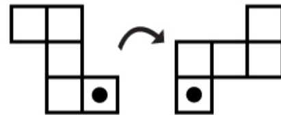
ROTATION
