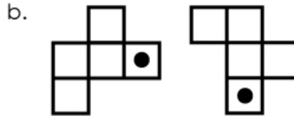
rotation
