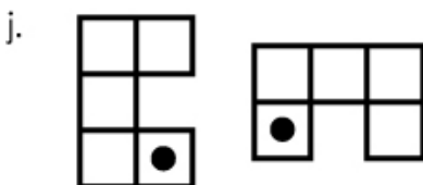
rotation
